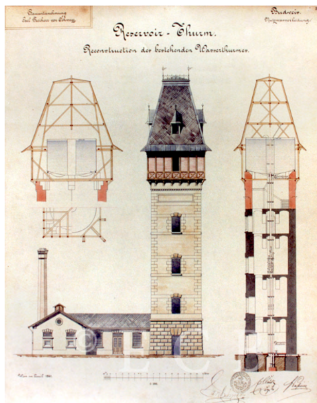
Obrázek 2: Plány vodárenské věže z roku 1881. SOkA. Zdroj: https://www.encyklopedie.c-budejovice.cz/clanek/vodarenska-vez
